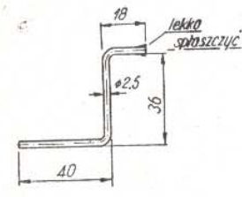
Rys. 13. Łaska hokejowa
