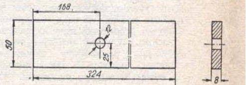
Rys. 4. Listwa boczna
