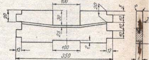
Rys. 3. Listwa czołowa
