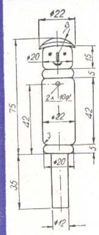
Rys. 11 Gracz
