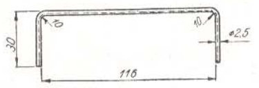
Rys. 8. Klamerka
