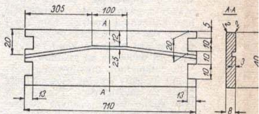
Rys. 2. Listwa boczna
