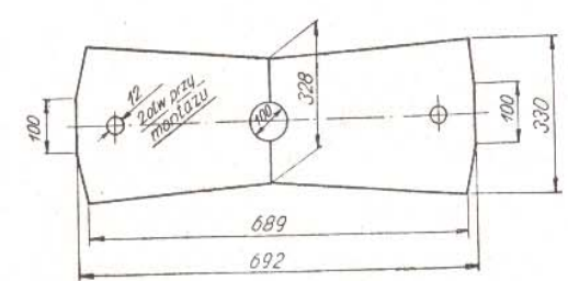
Rys. 10. Bieżnia
