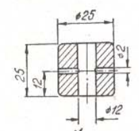
Rys. 12. Pokrętko
