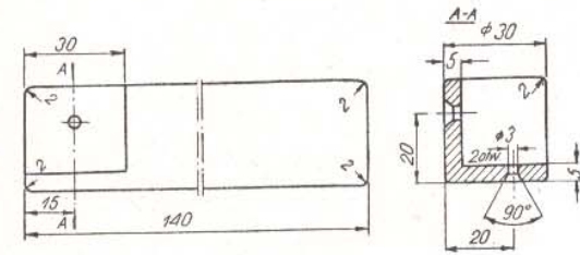
Rys. 6 Moźka
