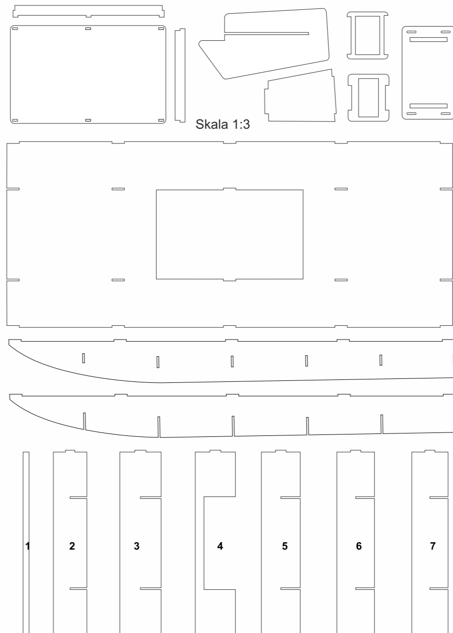
Podstawowe elementy konstrukcji modelu łodzi bagiennej MT-14
