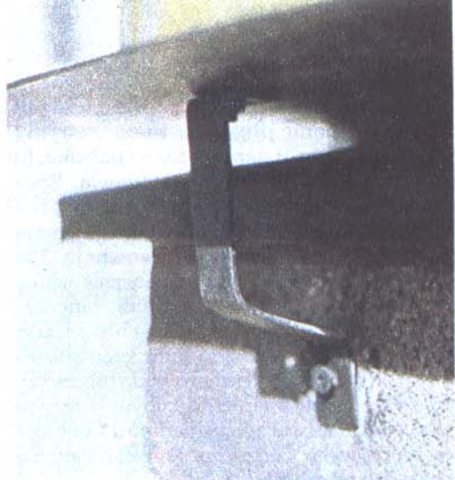
Sposób mocowania parapetu
