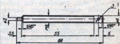
Rys. 3. Śruba
