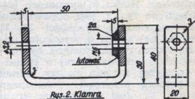
Rys. 2. Klamra
