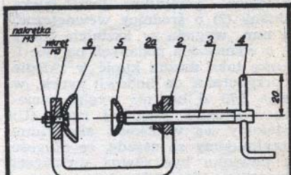
Rys. 1. Zgniatacz do orzechów
