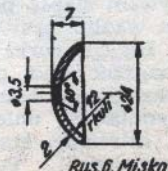
Rys. 6. Miska
